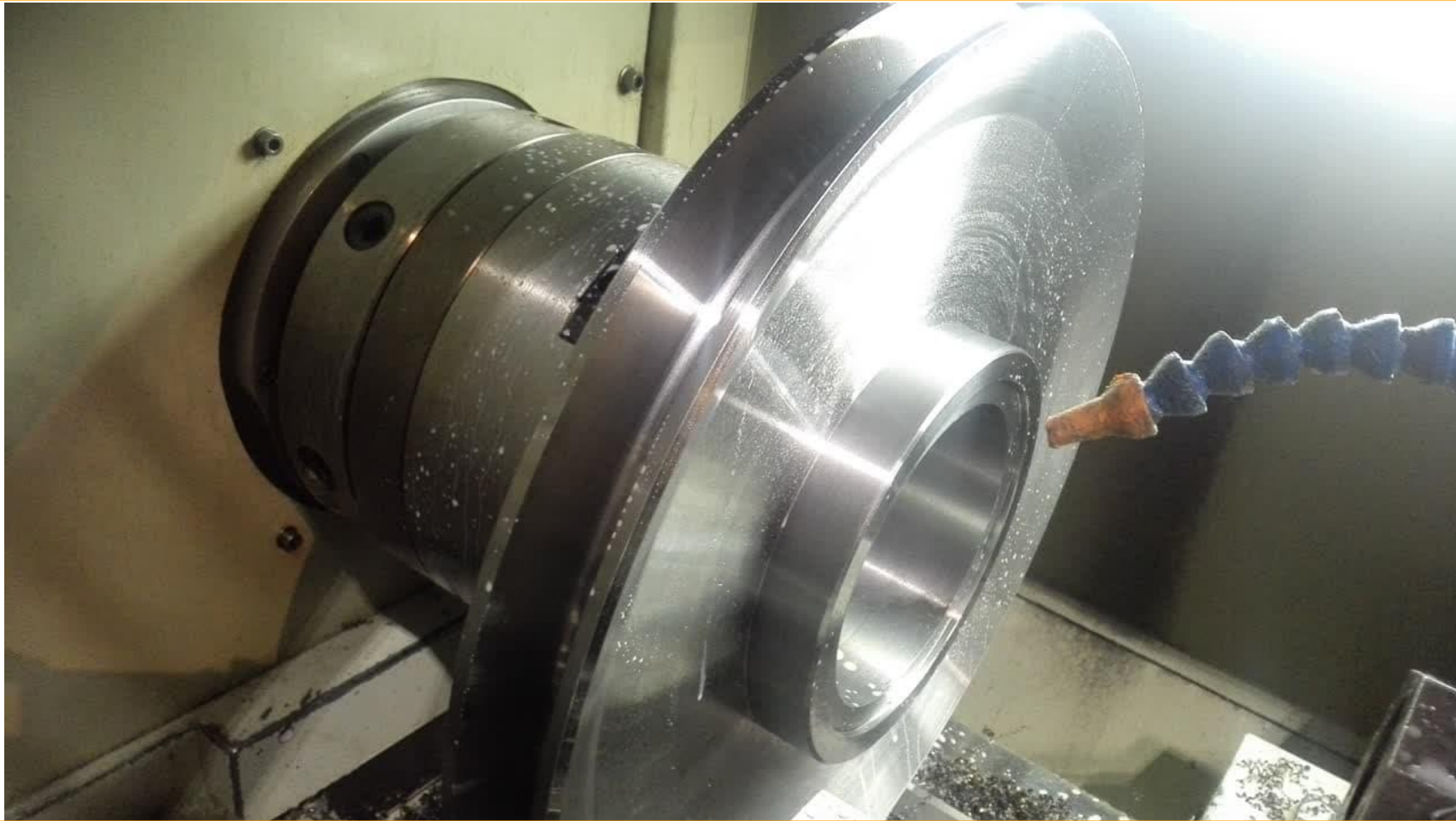
ساخت پولی های بزرگ فولادی جرثقیلهای بلند شرکتهای فولادی
